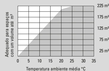
Adequação do DH 15 para manutenção do estado higrométrico de espaços
