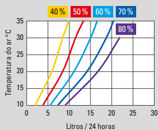
Capacidade de desumidificação DH 15
